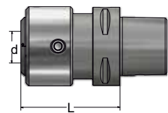
DIN ISO 26623-1
