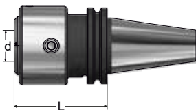
DIN 69871
